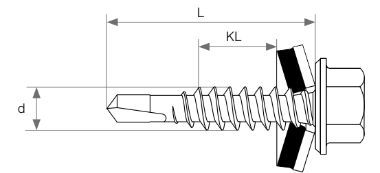
Abb. Selbstbohrende Schrauben - Aufbau
