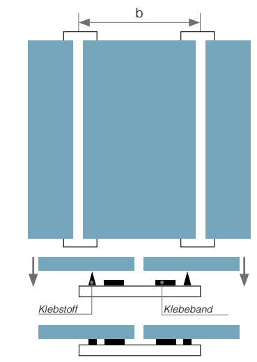
Beispiel für eine Einfeld Befestigung
