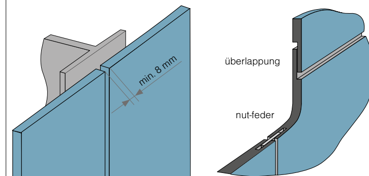
Abb. 0. Offenes Fugensystem
