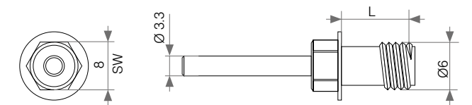
Abb. Nietschraube TU-S6,0x9 - Konstruktion und Abmessungen (mm)(mm).
