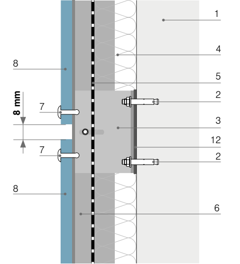
Abb. Schnitt B-B Profil-Verbindungsstück
