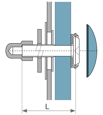
Abb. Aufbau und Abmessungen der Balkonschraube
