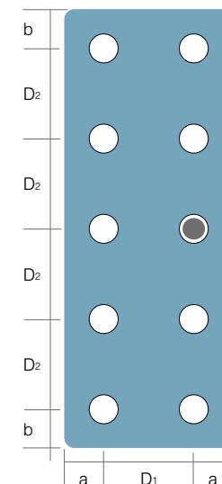
Fig. Einfeld-Befestigung
