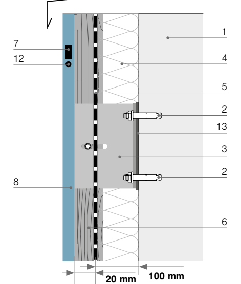
Abb. Schnitt F-F Oberer Teil der Wand mit Abschlussrahmen
